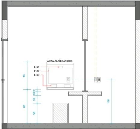
VISTA FRONTAL DA SALA ESCALA 1:25
